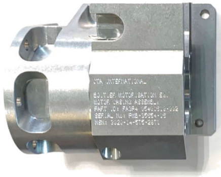
BOITIER MOTORISATION
